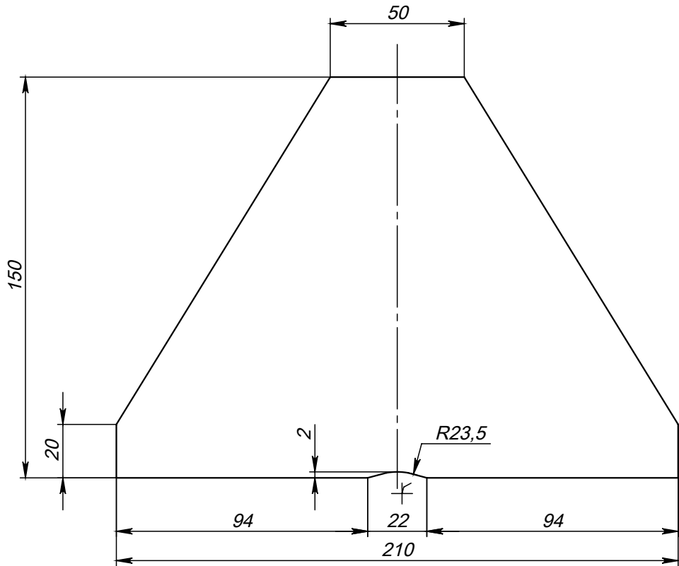
Поз.1 (Корпус) развертка
